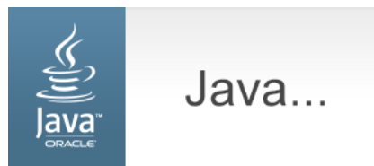
Рис. 11. Запуск Java
